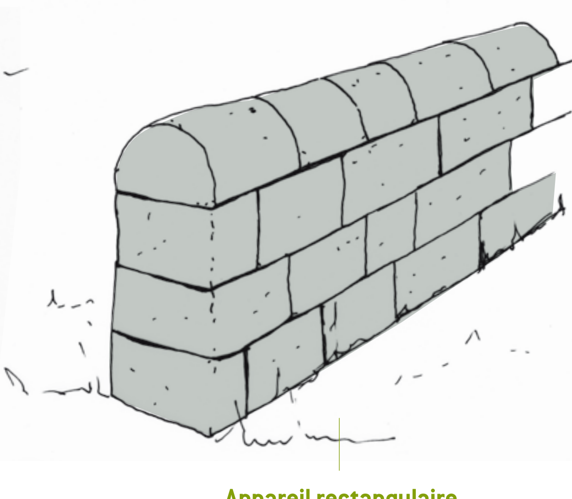
Appareil rectangulaire Couronnement en pierres arrondies ou « chaperon »
