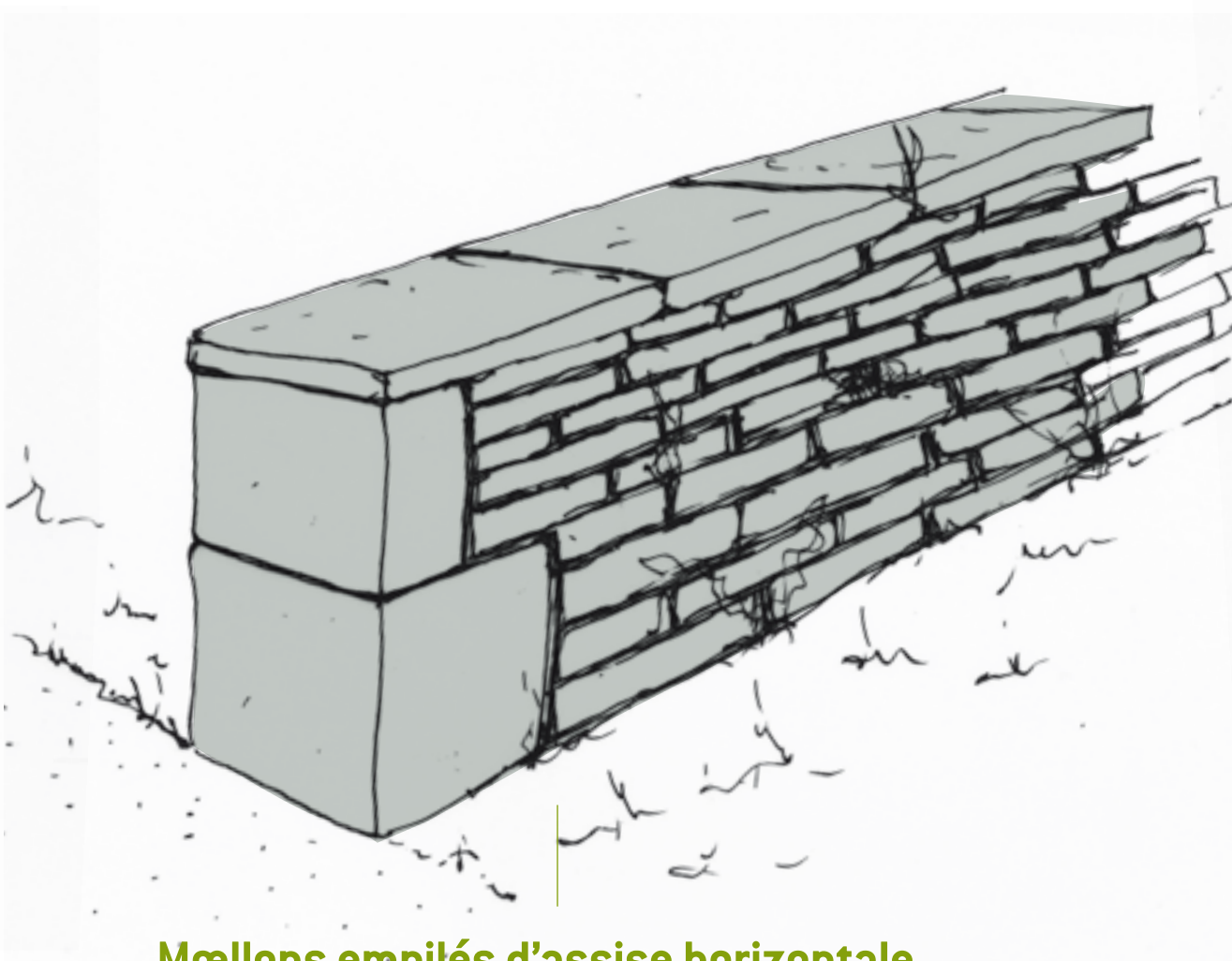
Mœllons empilés d'assise horizontale Couronnement en pierres plates
