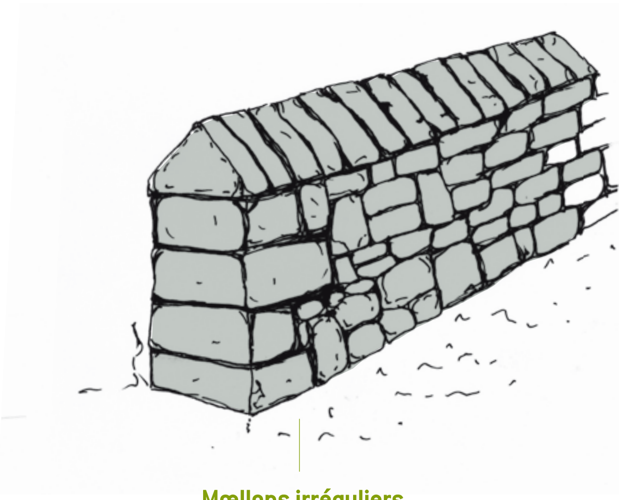
Mœllons irréguliers Couronnement en épis ou « râteau »
